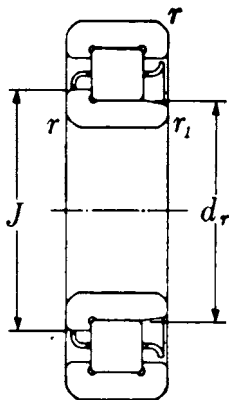
NJ3
