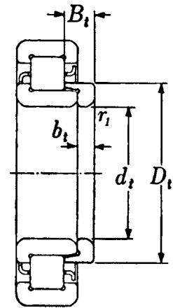
(NH2=NJ2+HJ2)
