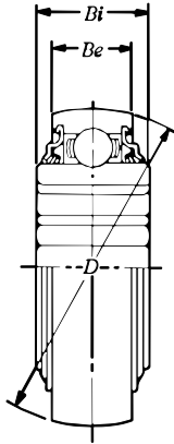
TYPE 2...V2
